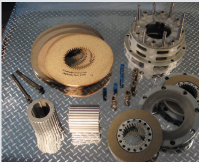
Éléments d'embrayage
